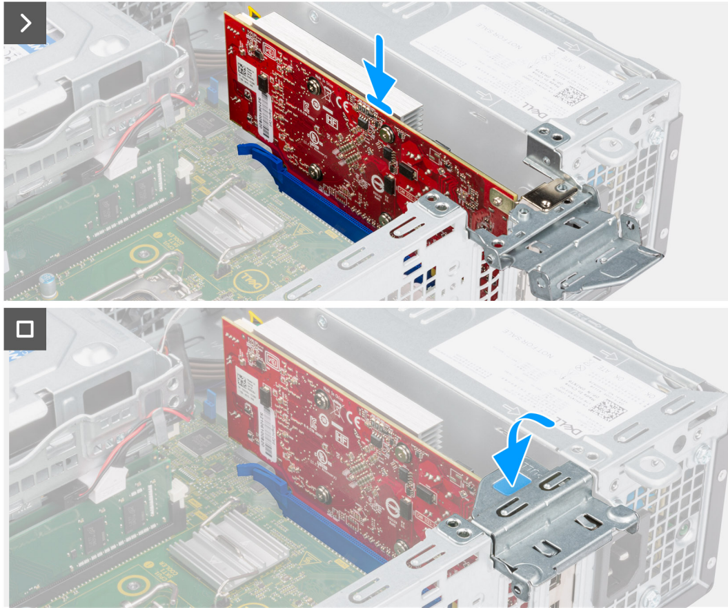
Ilustración 30. Instalación de la tarjeta gráfica
