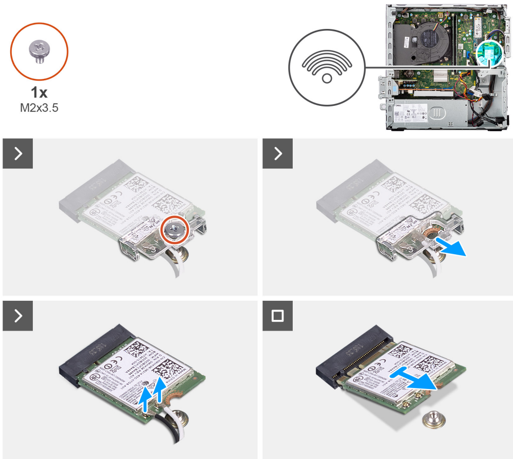
Ilustración 27. Extracción de la tarjeta inalámbrica
