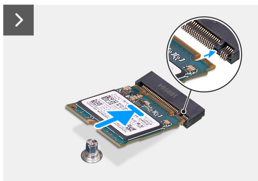
Ilustración 18. Instalación de las unidades de estado sólido M.2 2230
