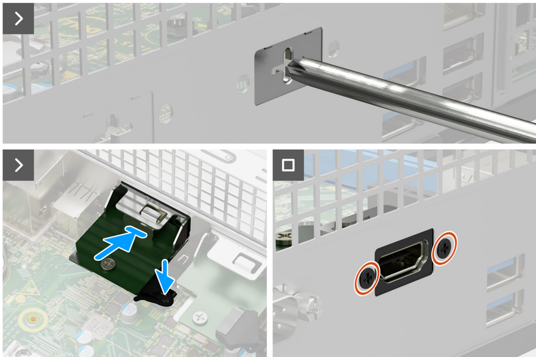
Ilustración 55. Instalación del módulo de HDMI
