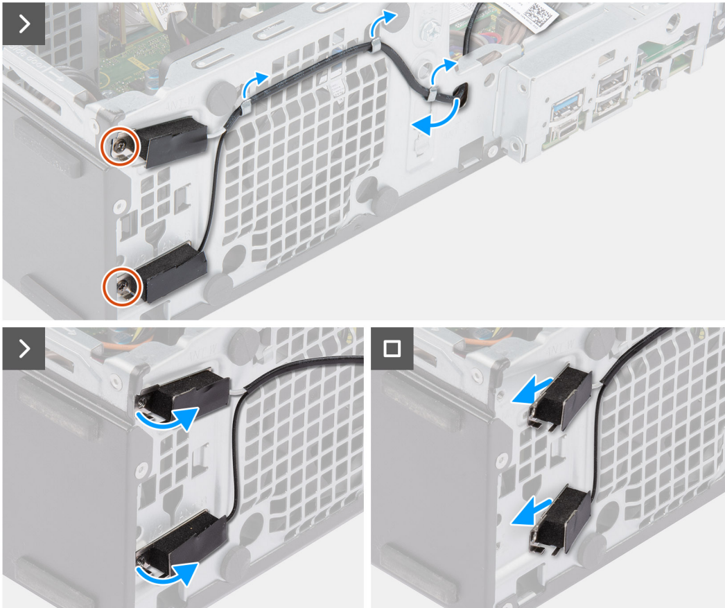
Ilustración 37. Extracción del módulo de la antena interna
